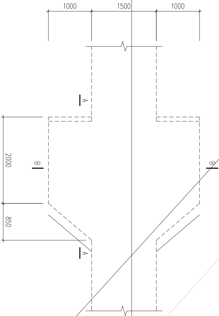
中墩牛腿平面布置图
